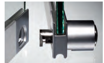
En el mecanismo patentado de pestillo de seguridad Secura, un bulón en forma de L integrado en la hoja delantera se encaja en el cerradero de la hoja posterior, evitando así la separación forzosa de las dos hojas. (A)
